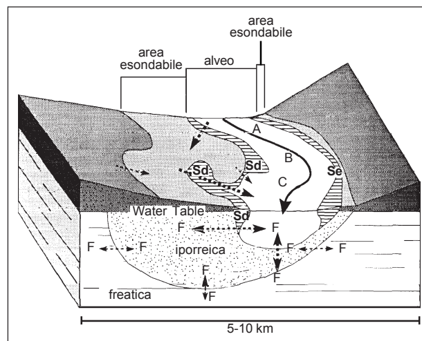
Fig. 2 - Schema dell'ambiente fluviale e ripario visto nelle 3 dimensioni spaziali (da STANFORD et al. 1996, modificato).
