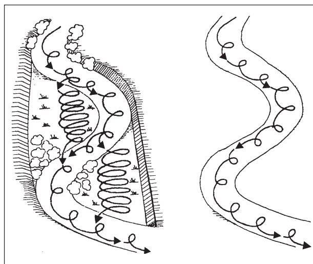
Fig. 3 - Schematizzazione della spiralizzazione dei nutrienti in un fiume naturale e in un corso d'acqua regolato e incanalato tra gli argini (tratto da PINAY et al. , 1990, modificato da BRAIONI, 1993).
