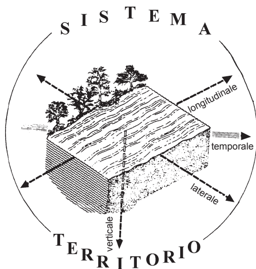
Fig. 1 - Visione pentadimensionale del sistema lotico (tratto da BOON 1992, modificato da BRAIONI et al. , 1998).
