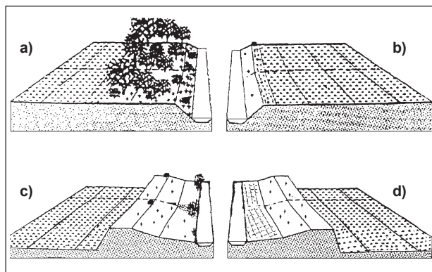
Fig. 4 - Schema rappresentativo: a) di aree riparie naturali alberate, b) prive di vegetazione, con le coltivazioni estese fino al fiume, c) di corsi d'acqua pensili con golena naturale, d) con golena coltivata. (tratto da PETERSEN et al., 1992, modificato da BRAIONI, 1993).
