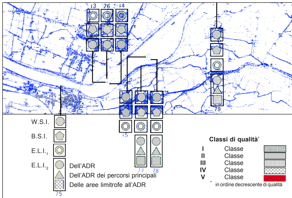
Mappa della qualità delle rive e delle aree riparie di un tratto del fiume Adige (Badia Polesine-Masi) (tratto da BRAIONI M. G. et al. , 1998).
