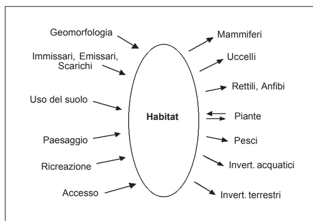
Fig. 8 - Il concetto di habitat come centro dell'ambiente fluviale naturale (tratto da HARPER et al. , 1995, modificato da DE FRANCESCO, 1996).
