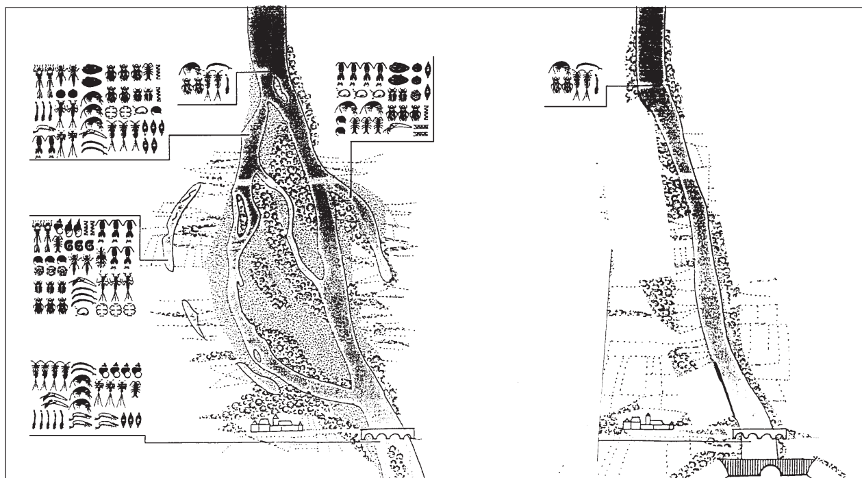
Fig. 5 - Esempio schematico sull'efficienza di ritenzione operata dal macrobenthos in un fiume naturale e in uno regolato con perdita di meandri, isole, rami laterali (tratto da WWF, 1990 modificato da BRAIONI 1993).
